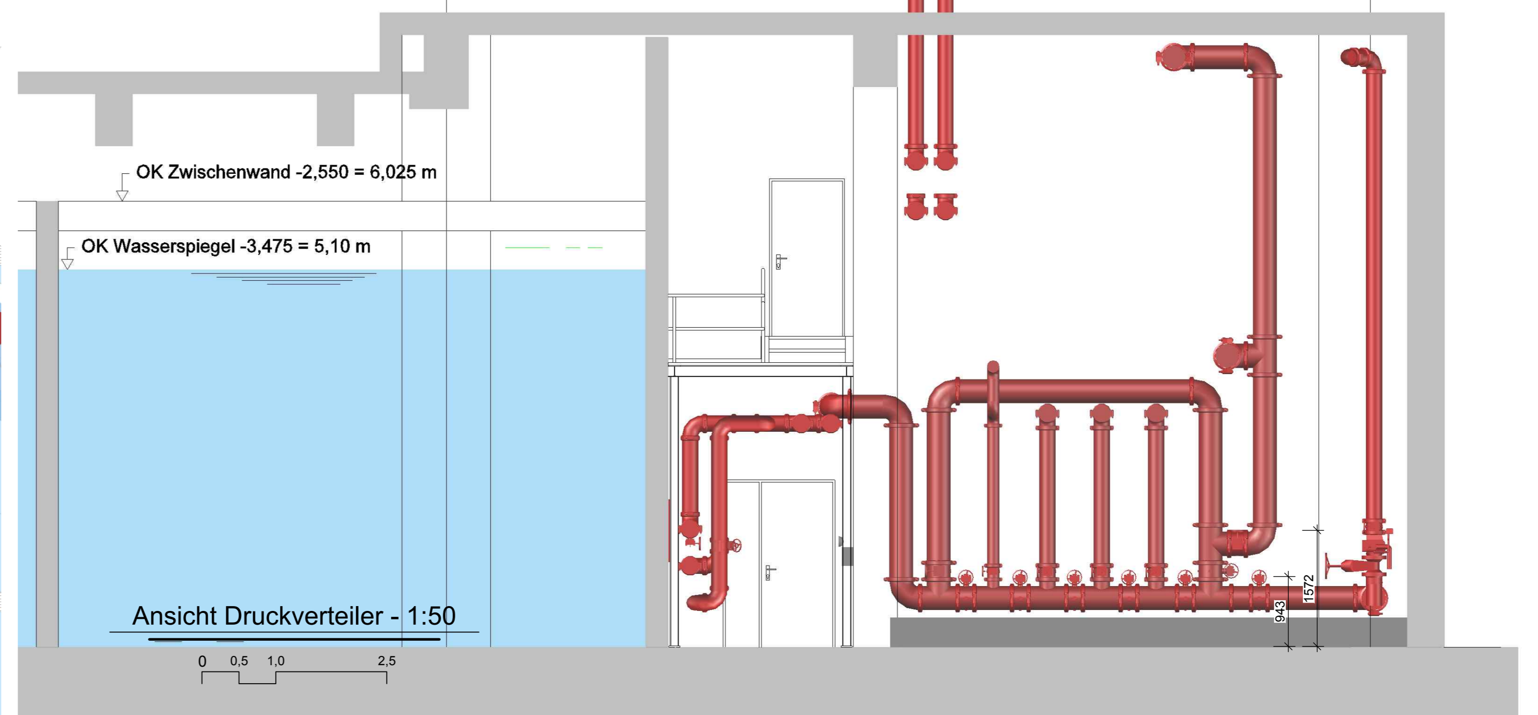
Ansicht E-Pumpe - 1:50
