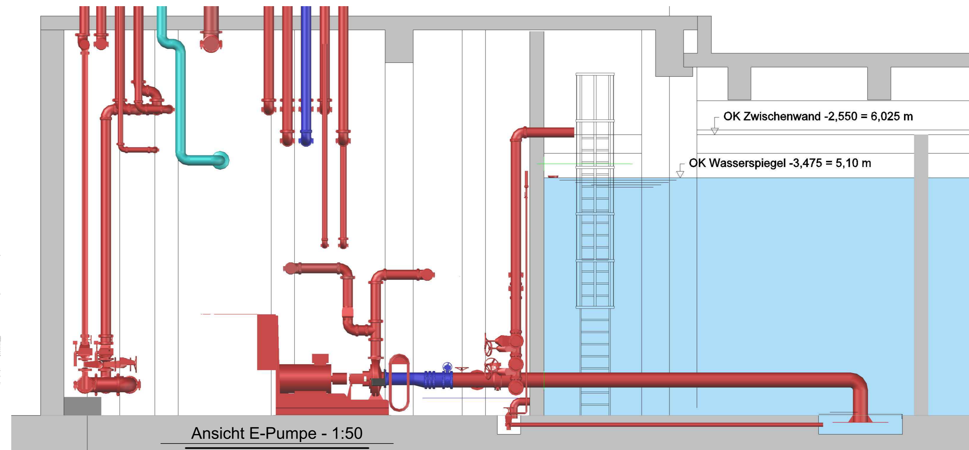
Ansicht D-Pumpe und DLWB - 1:50
