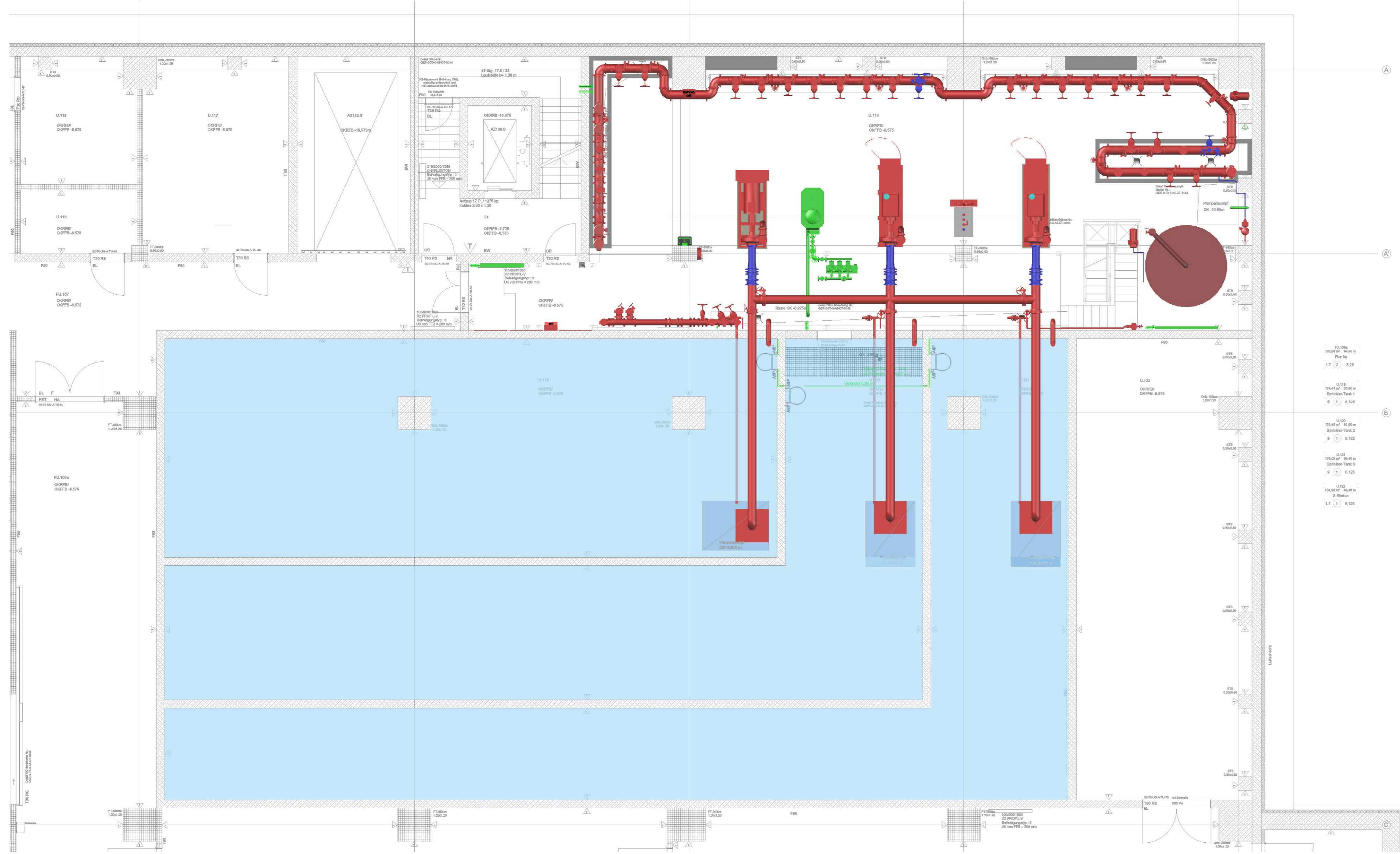
Grundriss - 1:100
