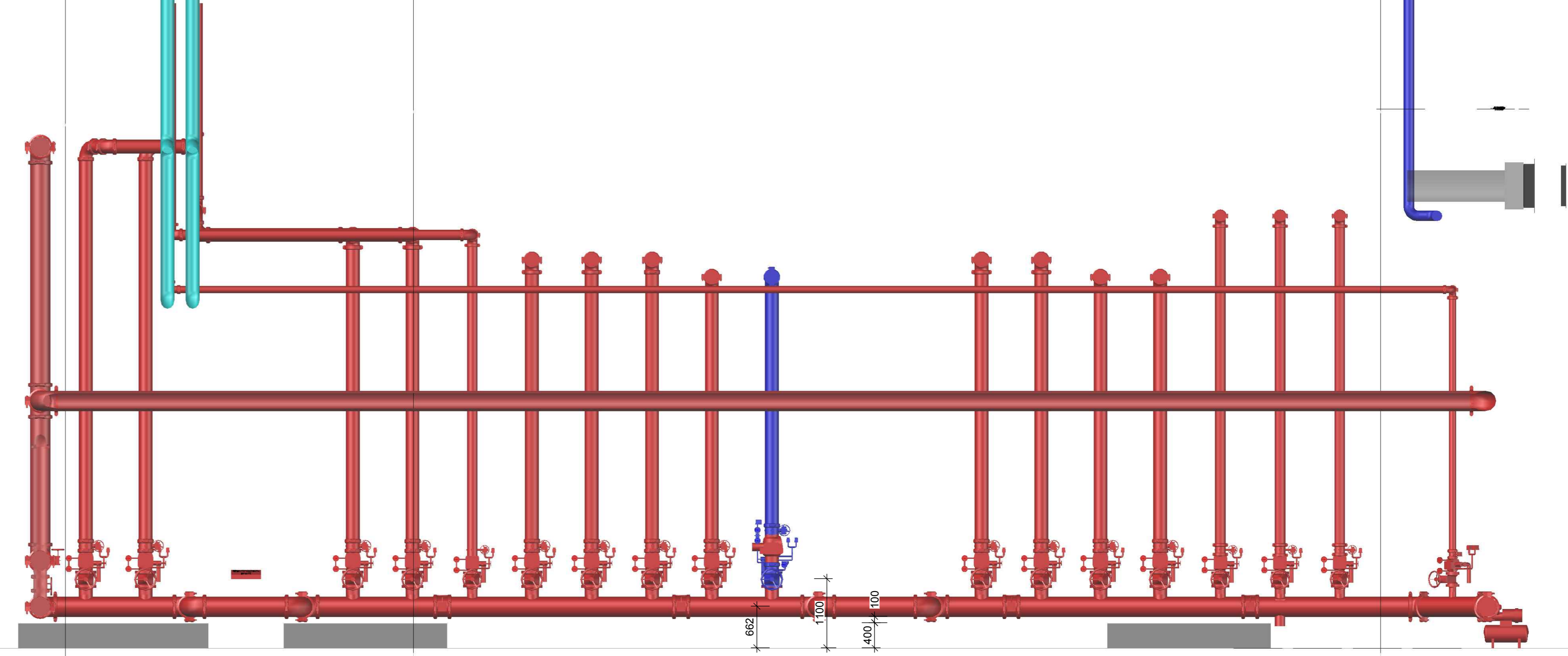
Ansicht Sprinklerverteiler - 1:50
